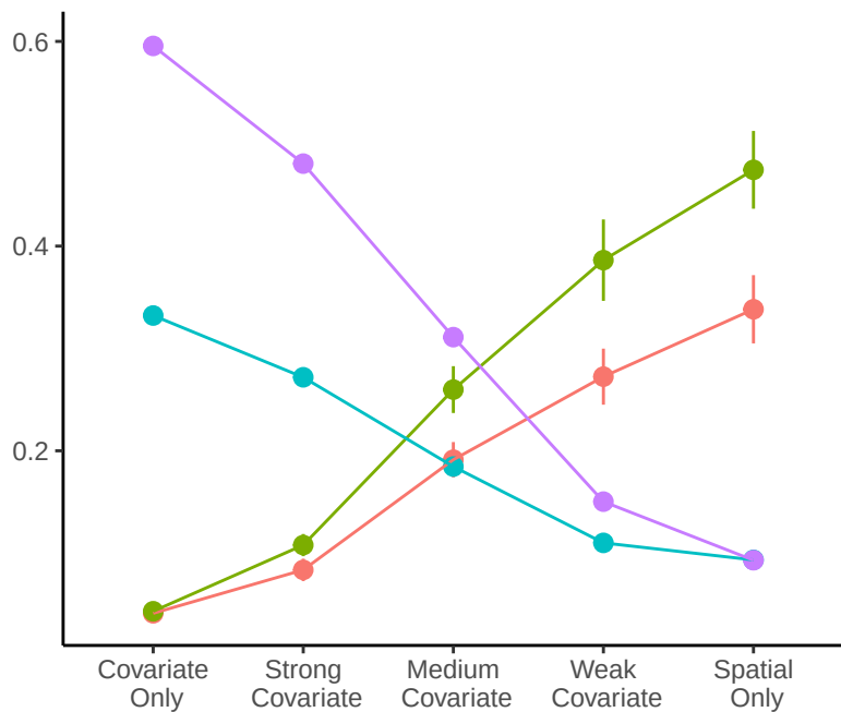
Interval Width
